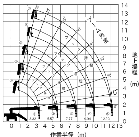
作業範囲図
